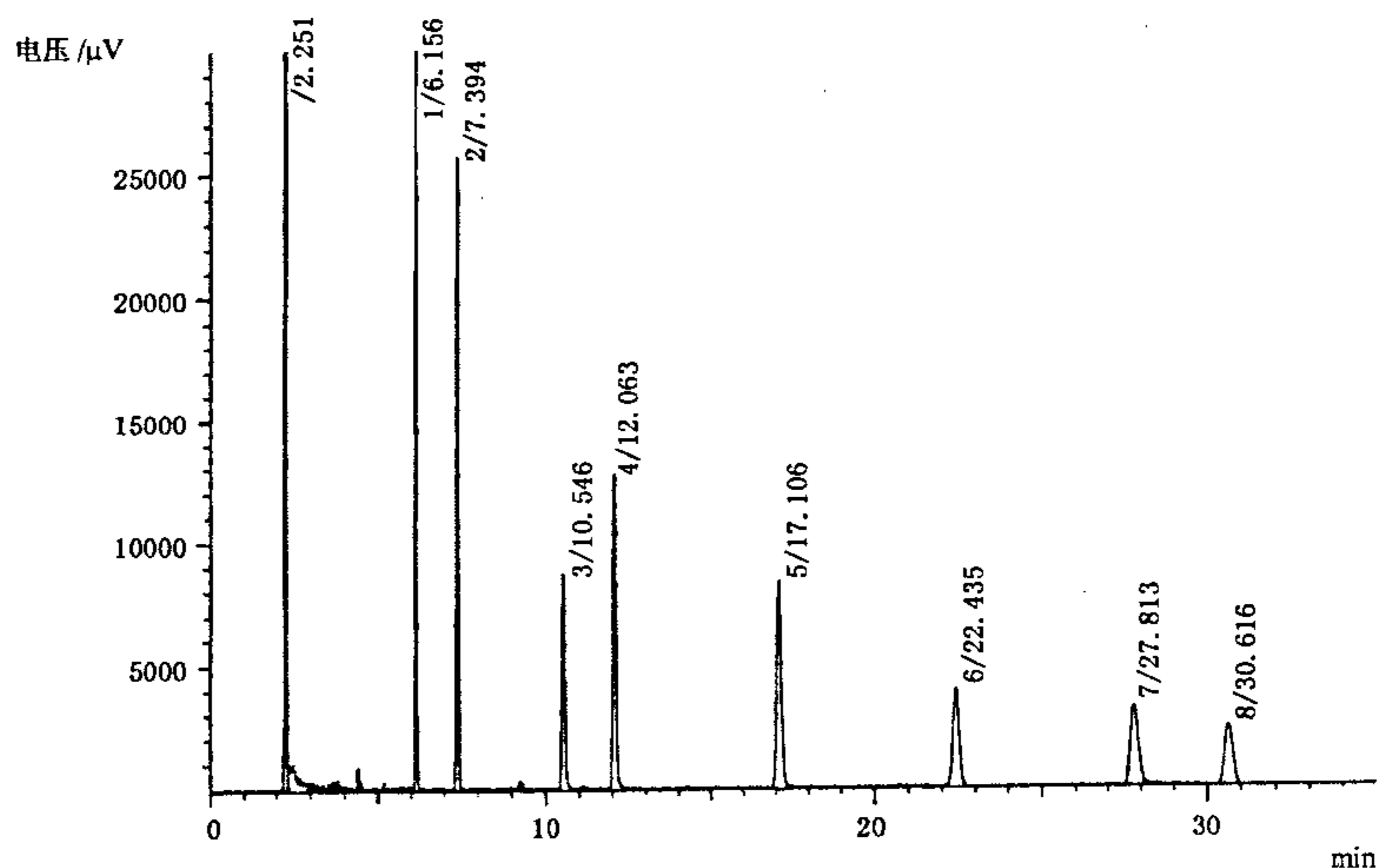
图 2 标准色谱图
